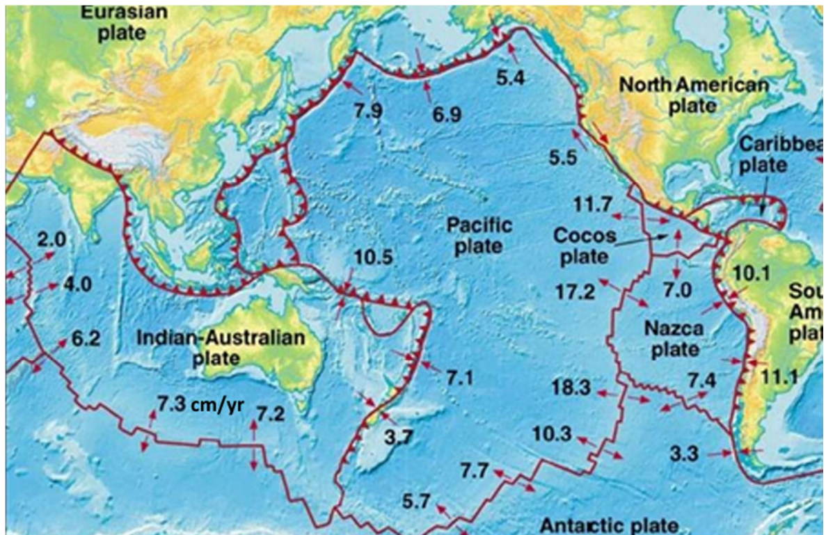
Gambar 4. Ilustrasi sistem tektonik lempeng
